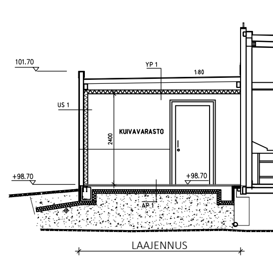
LEIKKAUS A-A
